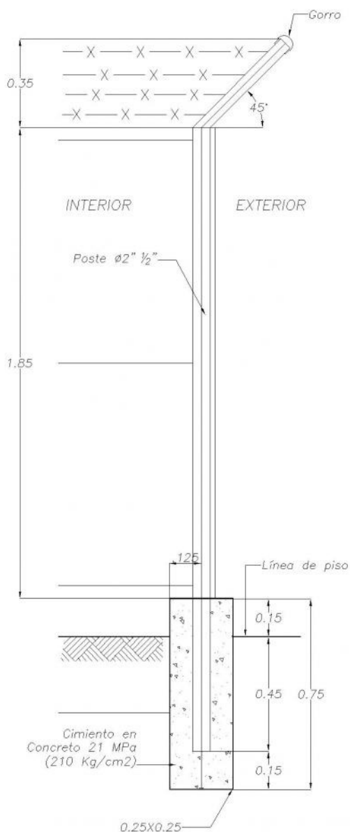
CORTE SOBRE EL TUBO
