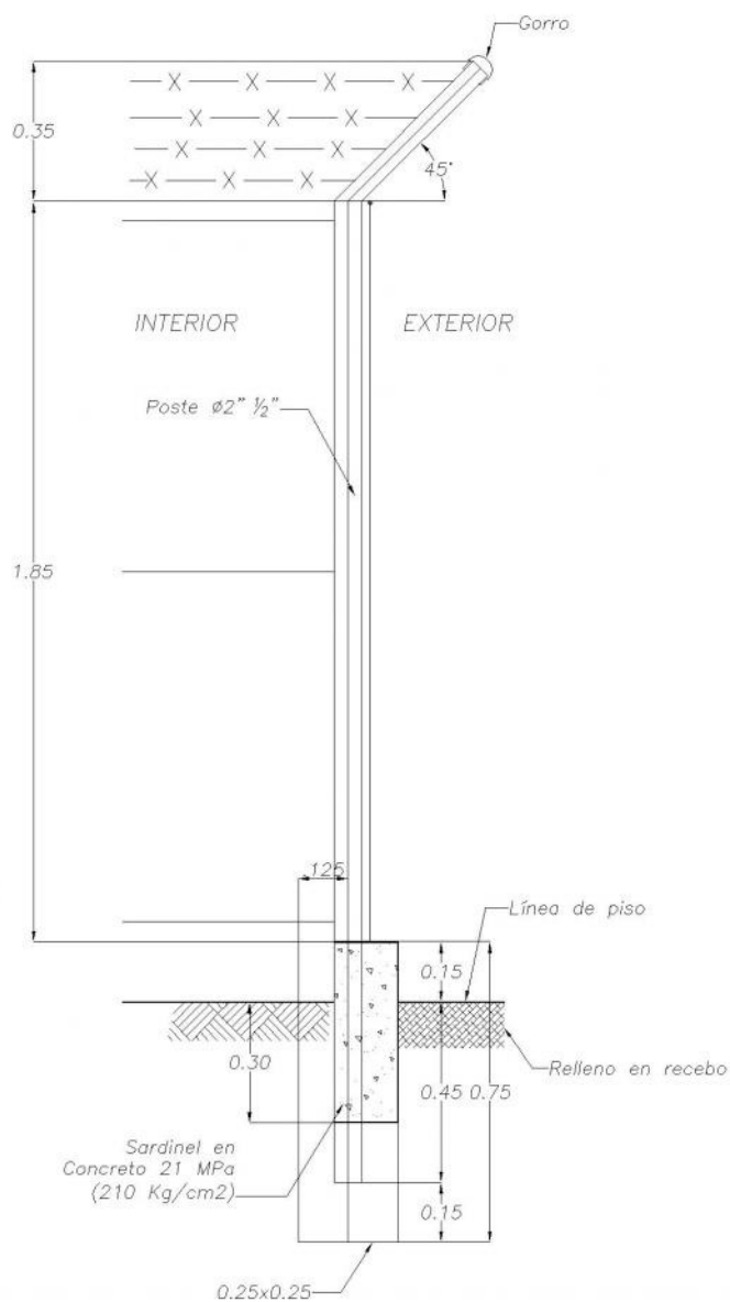
CORTE SOBRE LA MALLA
