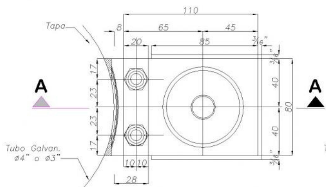
DETALLE 1 - PLANTA
