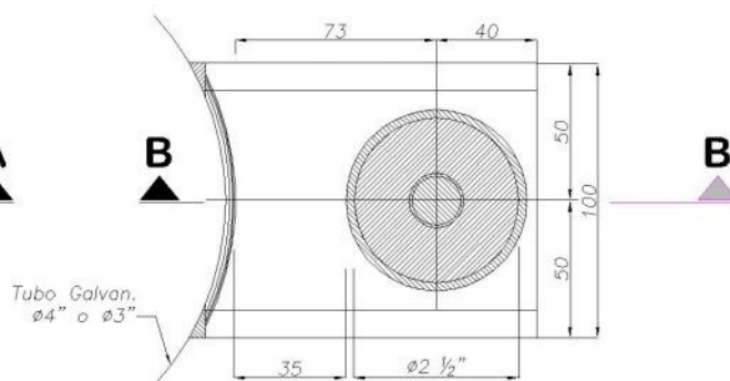
DETALLE 2 - PLANTA
