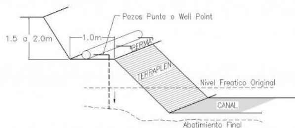
FIGURA 1 POZOS PUNTA O WELL POINT
