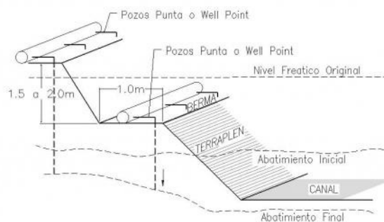
FIGURA 3 HILERAS DE PUNTAS DE WELL POINT ESCALONADAS
