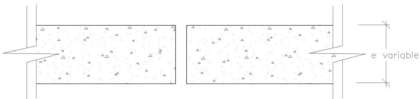
JUNTA PLANA DE DILATACION PARA PENDIENTES DE CUNETAS MENORES A 5%
