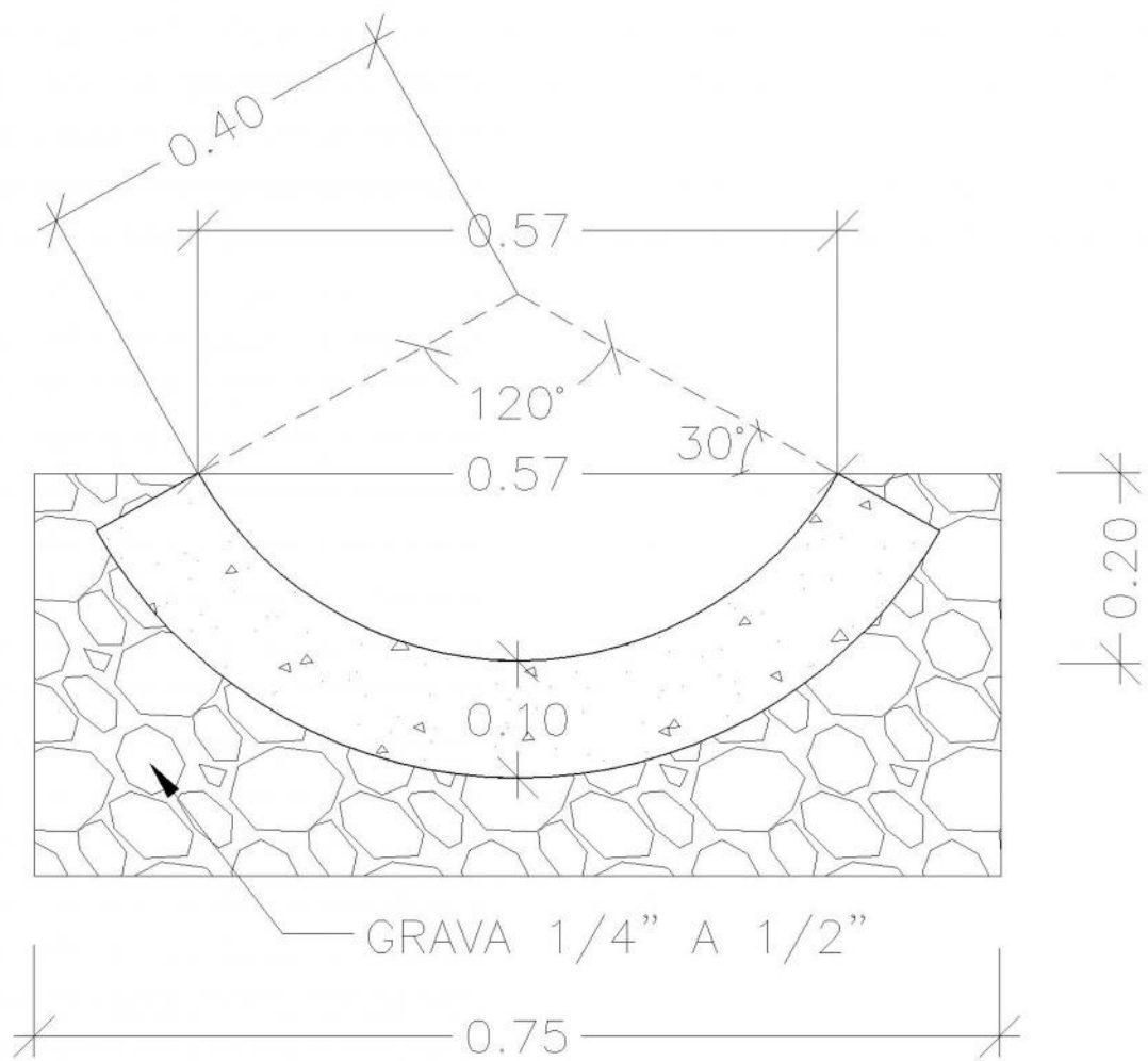
CUNETA SECCION SEMICIRCULAR
