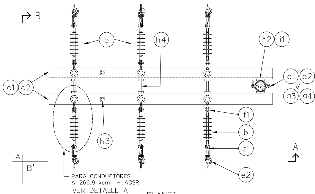
PLANTA
