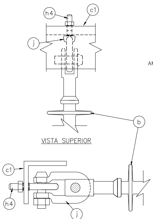
DETALLE A – VISTA LATERAL
