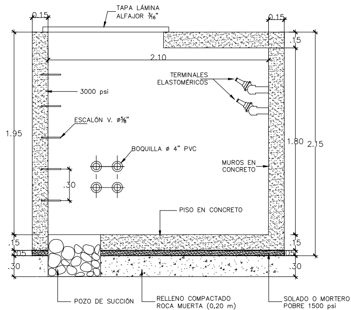
CORTE B-B'
