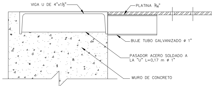
CORTE A-A'
