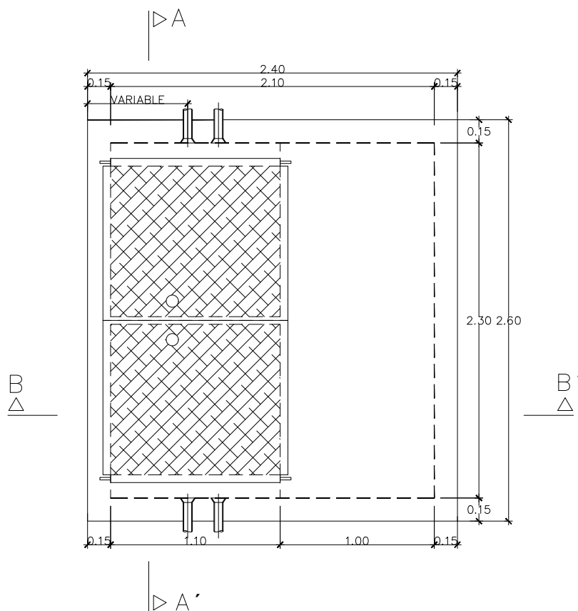
PLANTA ESC. 1:XX CÁMARA DE MANIOBRA TIPO B2 (2,50x2,60x1,80)
