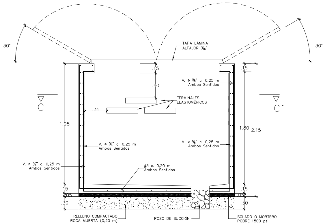
CORTE A-A'
