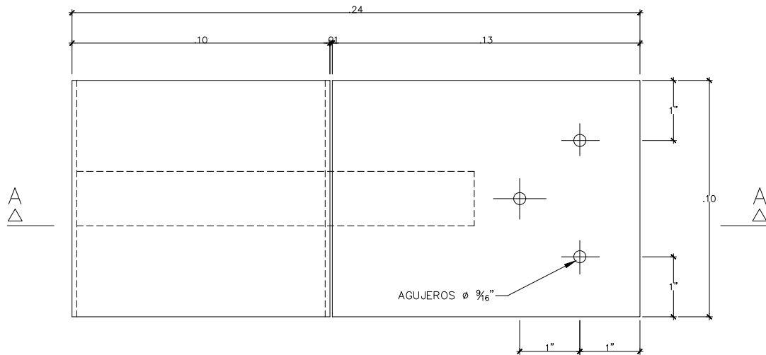
DETALLE DE BISAGRA
