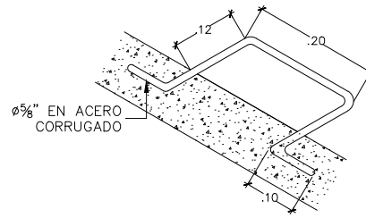
DETALLE DE ESCALONES
