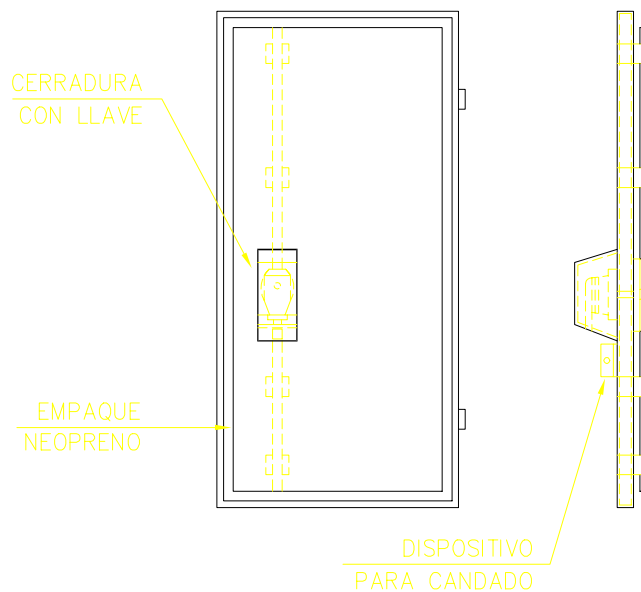
DETALLE "A" PUERTAS METALICAS
