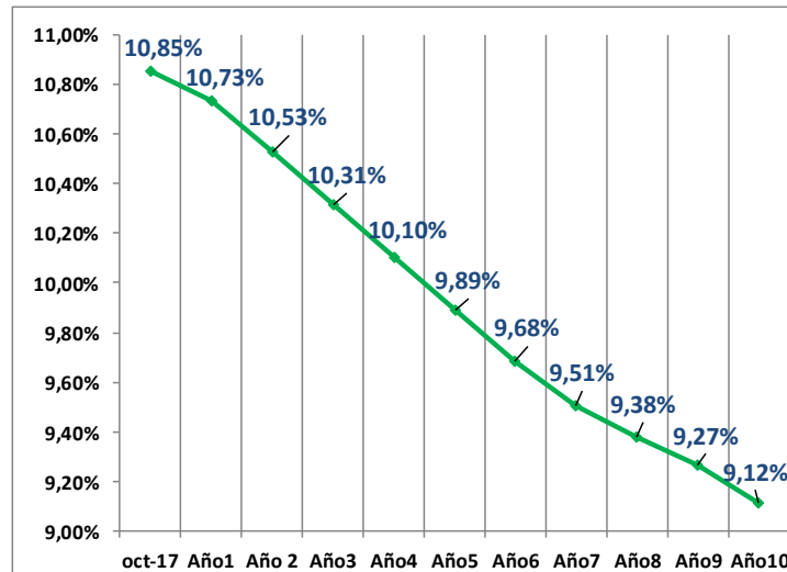
Senda de reducción de pérdidas de energía Índice de pérdidas totales IPT (%)
