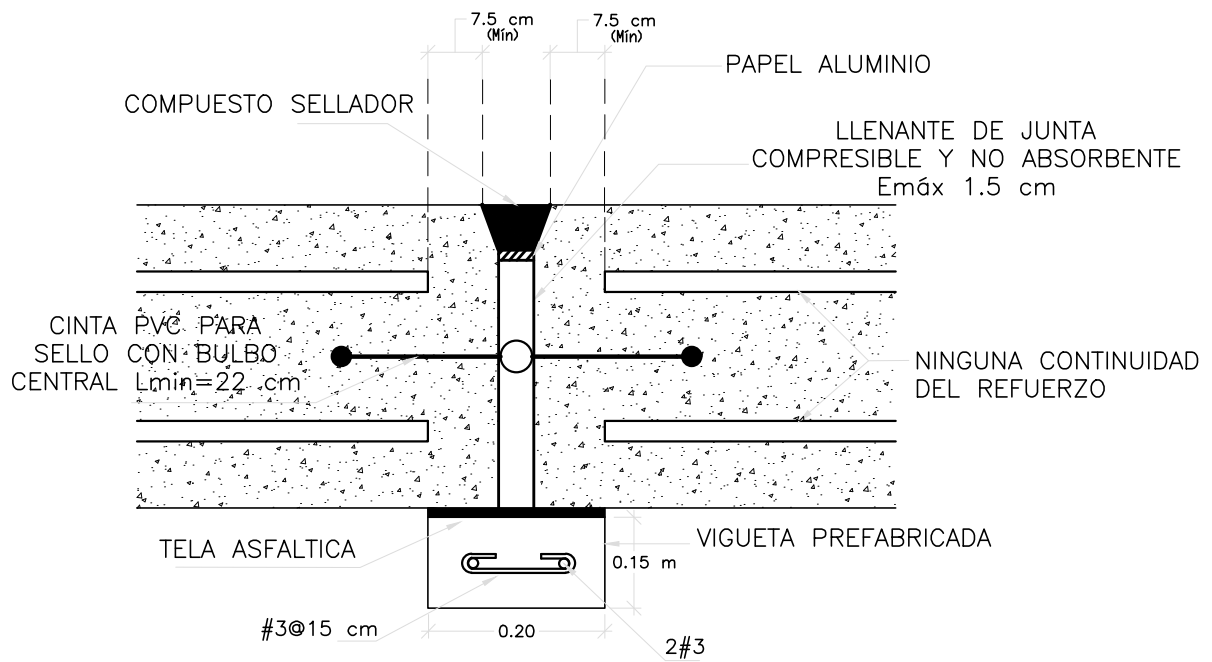
JUNTA DE EXPANSIÓN EN LOSA DE FONDO
