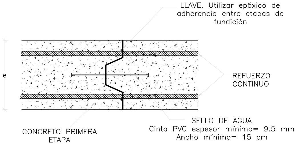
JUNTAS DE CONSTRUCCION CON LLAVE
