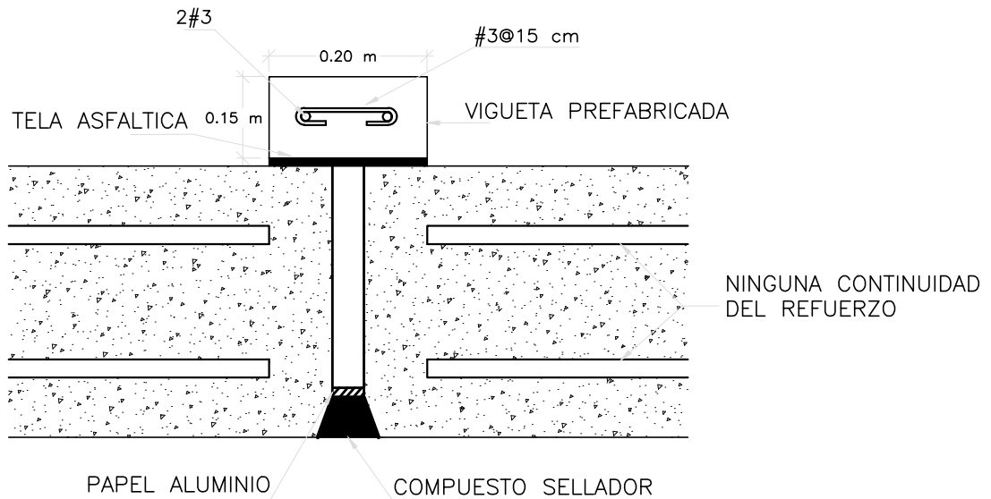
JUNTA DE EXPANSIÓN EN LOSA SUPERIOR
