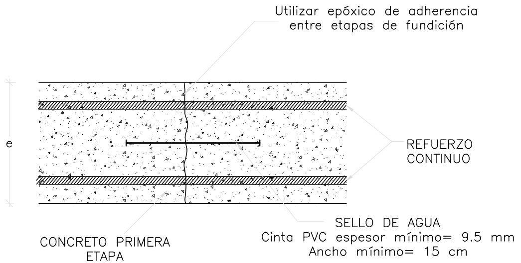
JUNTAS DE CONSTRUCCIÓN SIN LLAVE
